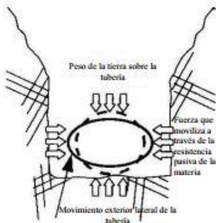
Fig. 3.1 Deflexión de la tubería.
